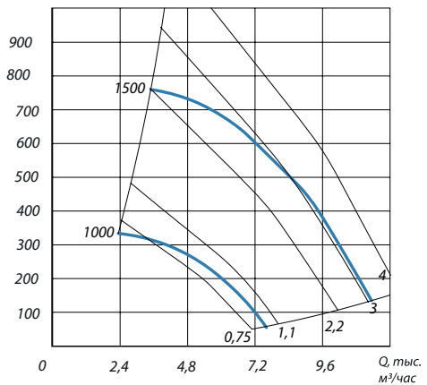
Р стат. Па ВРК.ВК.5,6
