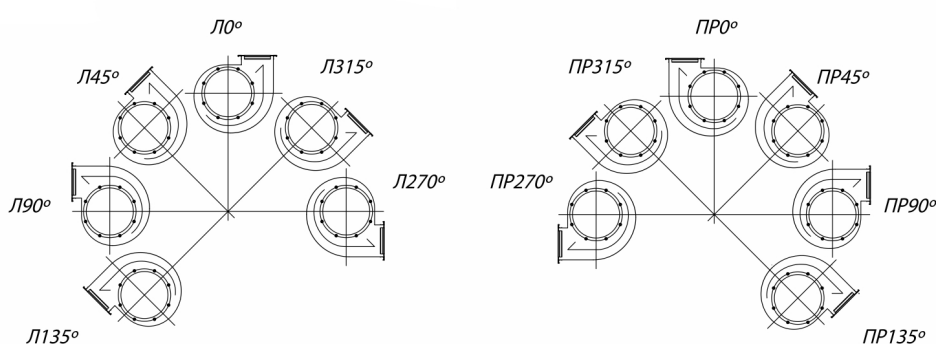
Положение корпуса вентилятора радиального ВР.80-75 (Вид со стороны всасывающего патрубка)
