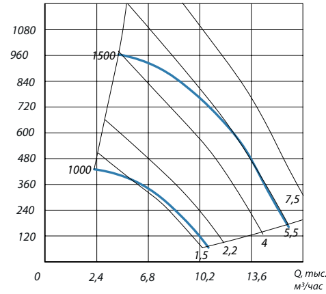
Р стат. Па ВРК.ВК.6,3
